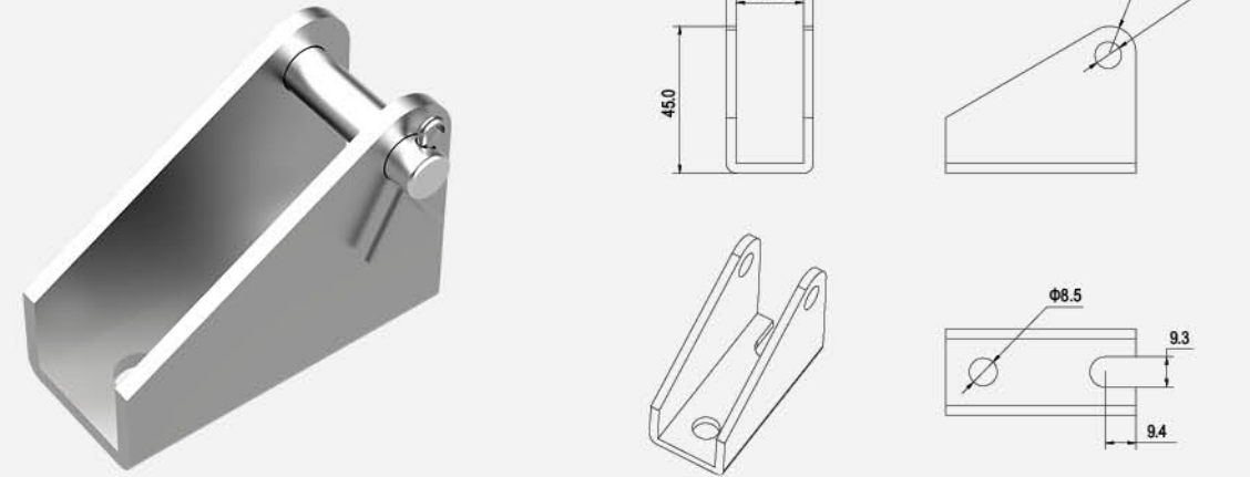
支架 U 型
